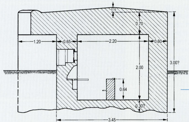
Schnitt A-A
